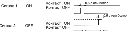
(В) Импульсный сигнал
